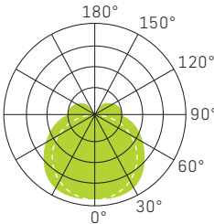
COURBE PHOTOMÉTRIQUE
