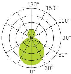
COURBE PHOTOMÉTRIQUE
